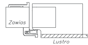
wariant 3 otwierany do wewnątrz ODW lustro od strony przeciwnej do zawiasów (A/Z)
