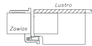
wariant 4 otwierany do wewnątrz ODW lustro od strony zawiasowej (Z)
