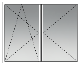
dwuskrzydłowe: rozwierne+uchylno-rozwierne, uchyln-rozwierne + rozwierne, uchyln-rozwierne + uchyln-rozwierne double-sashed: turn +tilt&turn, tilt&turn + turn, tilt&turn + tilt&turn
