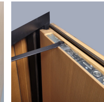
Verdeckter Türschließer
