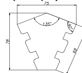
Łącznik kątowy 135°
