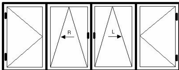
SŁUPEK STAŁY SŁUPEK RUCHOMY SŁUPEK STAŁY
